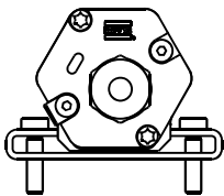
Kabelausgang P02
