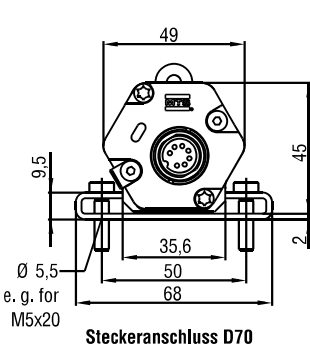
Steckeranschluss D70
